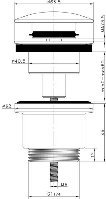
rysunek techniczny
