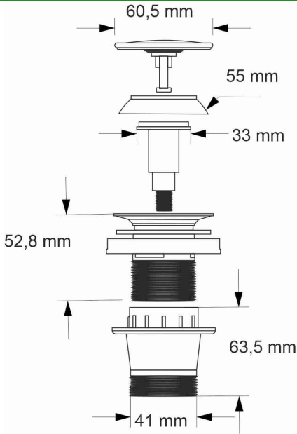
rysunek techniczny
