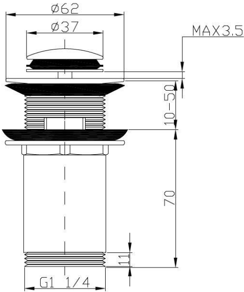
rysunek techniczny
