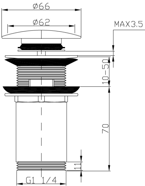
rysunek techniczny
