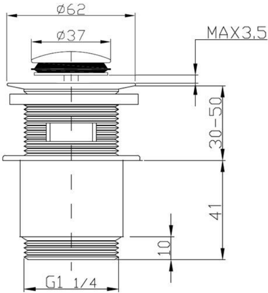
rysunek techniczny
