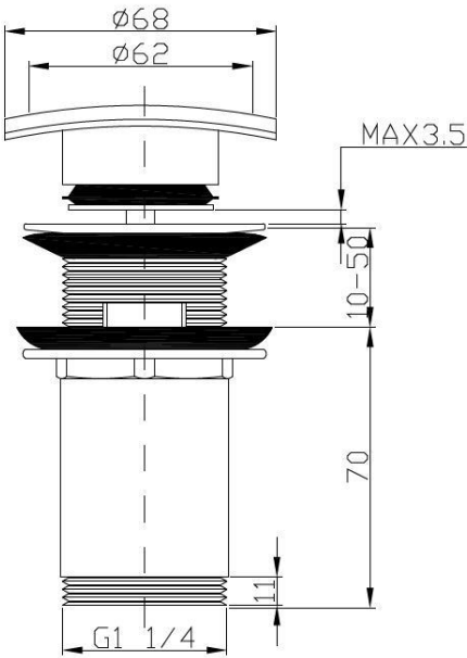
rysunek techniczny
