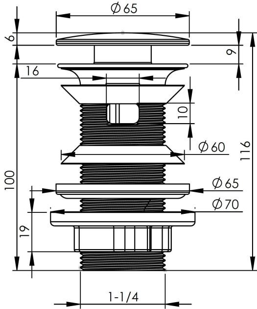
rysunek techniczny
