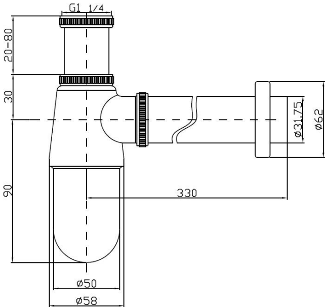
rysunek techniczny
