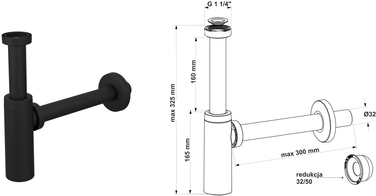
rysunek techniczny
