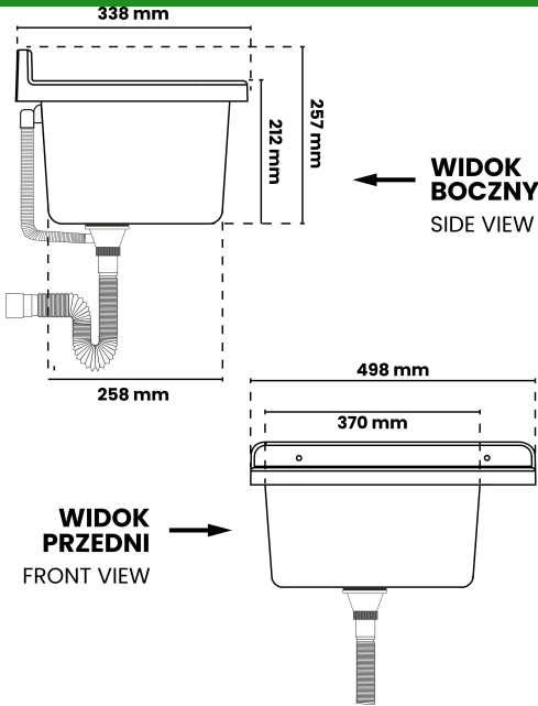
rysunek techniczny
